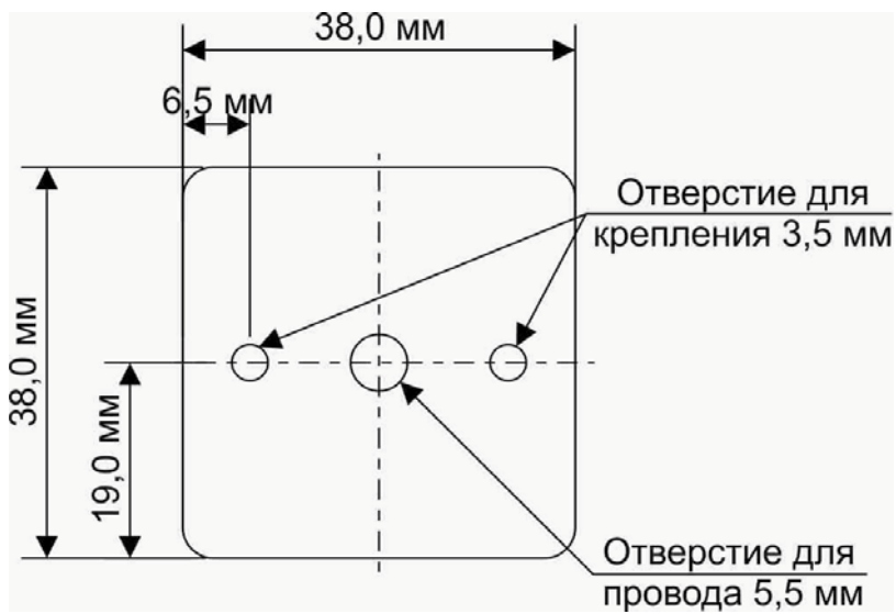
Рисунок 3 Установочные размеры устройства (основание)
