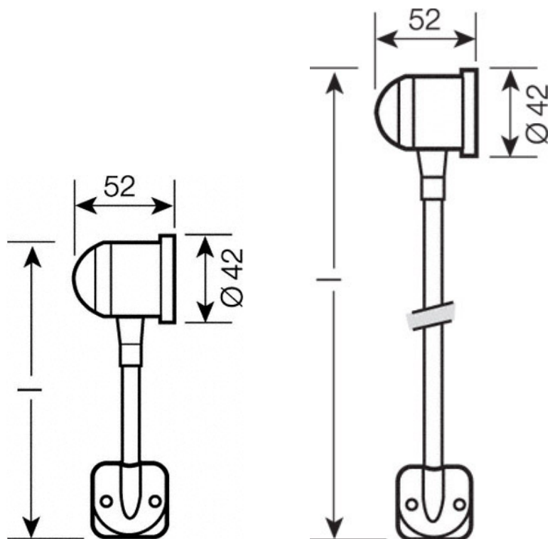
Рисунок 2 Габаритные размеры устройства
