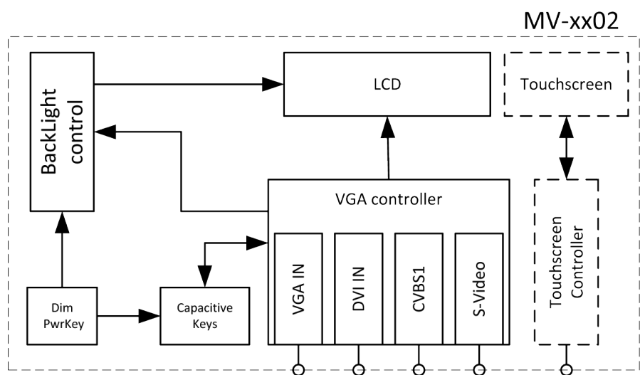
Функциональная схема
