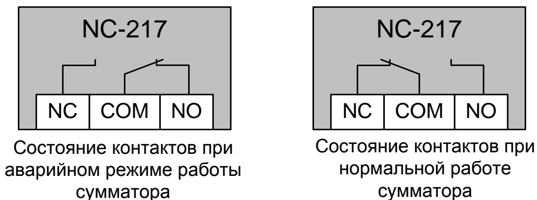
Рисунок 8. Состояние контактов релейного выхода «ALARM_OUT_AU-106».
