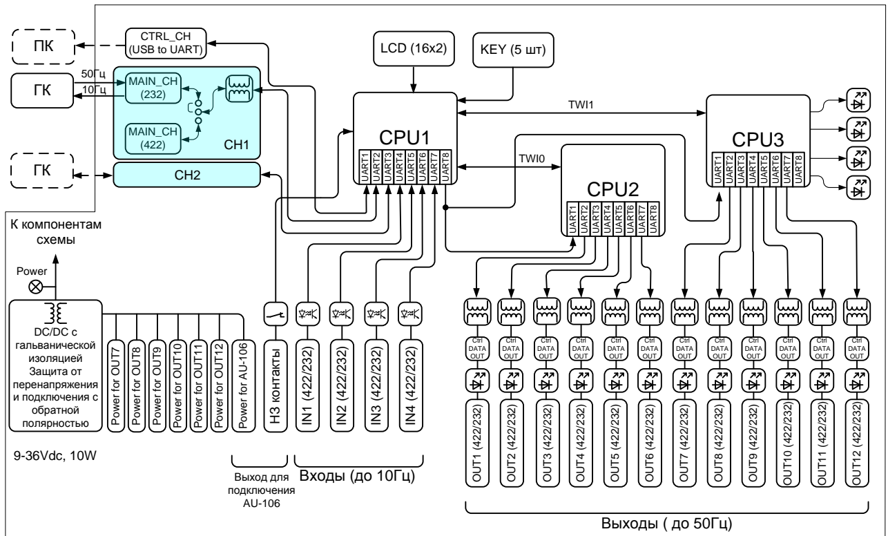
Рисунок 2. Структурная схема NC-217
