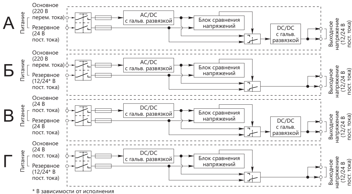
Функциональная схема БП-303
