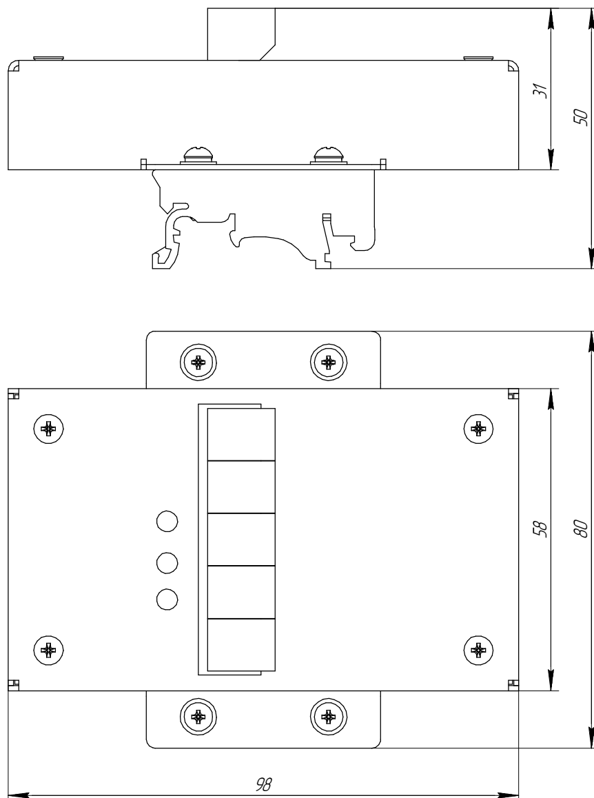
Габаритные и установочные размеры ПИ-104
