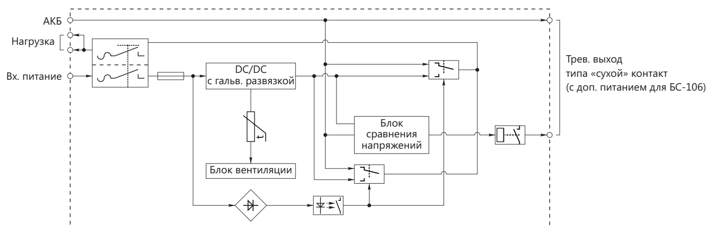
Функциональная схема БП-203-35, БП-203-40, БП-203-50, БП-203-60
