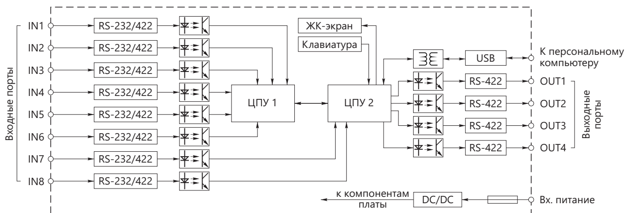
Функциональная схема СД-117
