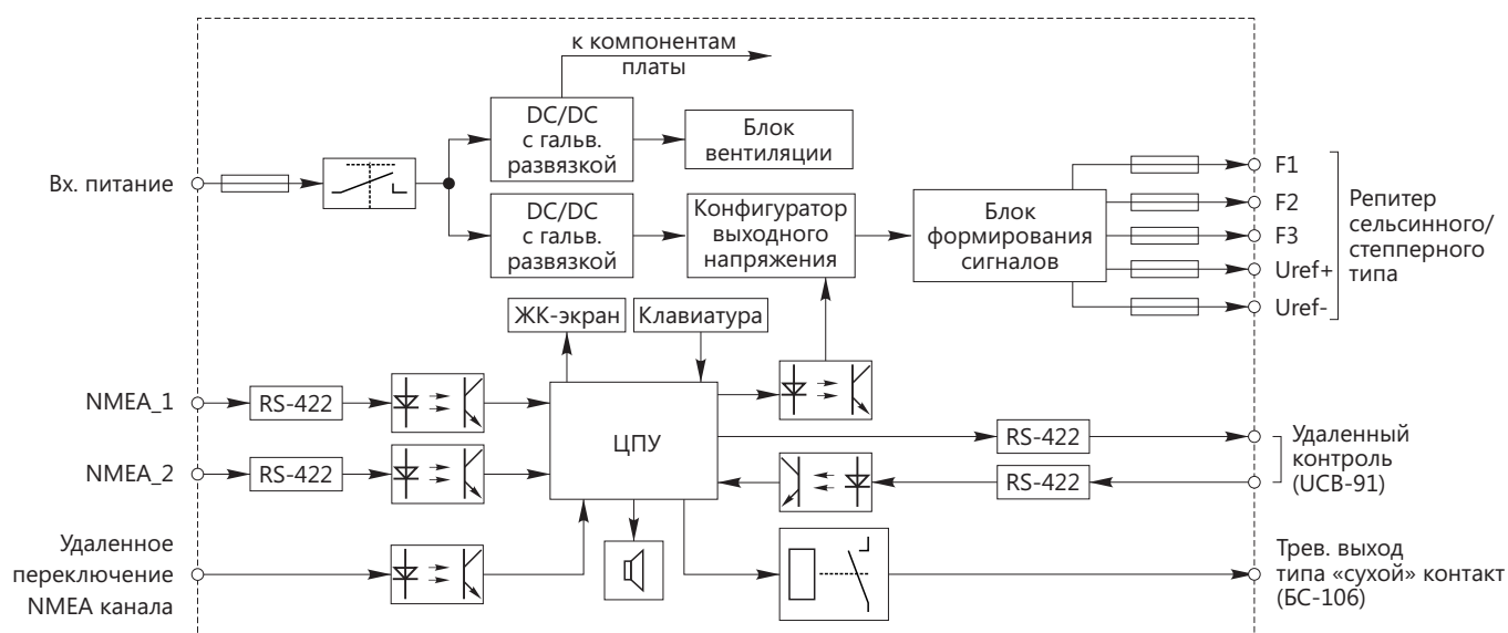
Функциональная схема ТКУ-109
