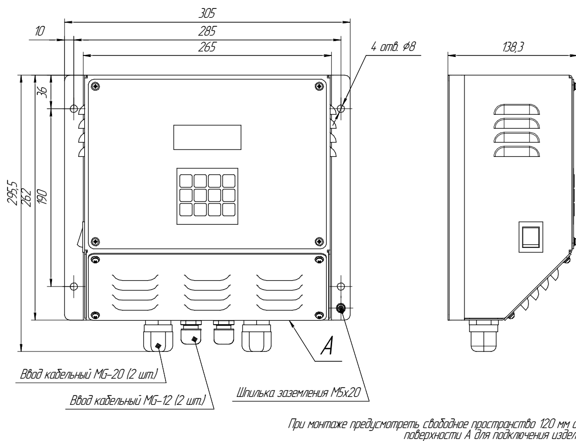
Габаритные и установочные размеры ТКУ-109
