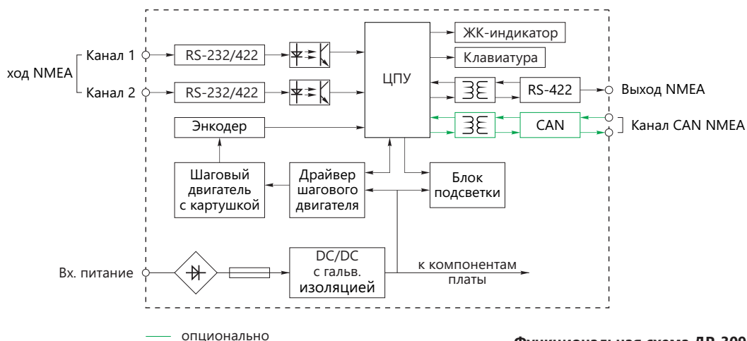
Функциональная схема ДР-309
