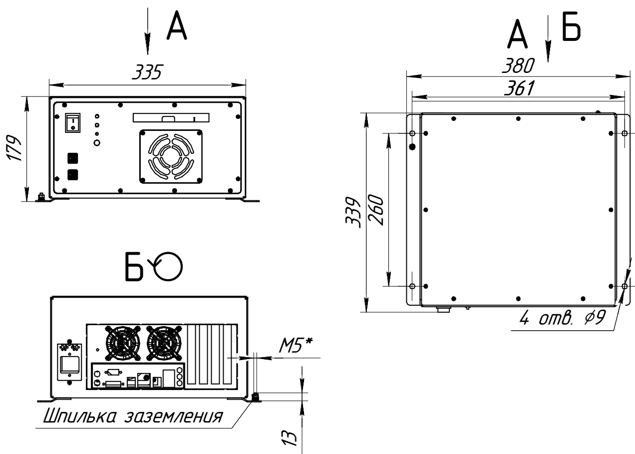
Габаритные и установочные размеры СБК-127
