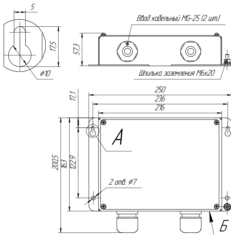
Габаритные и установочные размеры ФС-122
