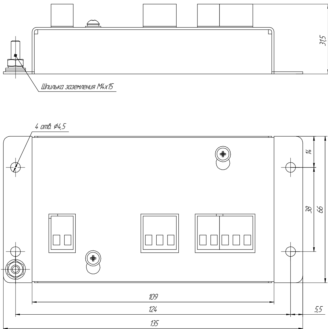
Габаритные и установочные размеры УПД-118
