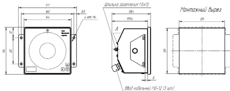
Габаритные и установочные размеры ДР-309
