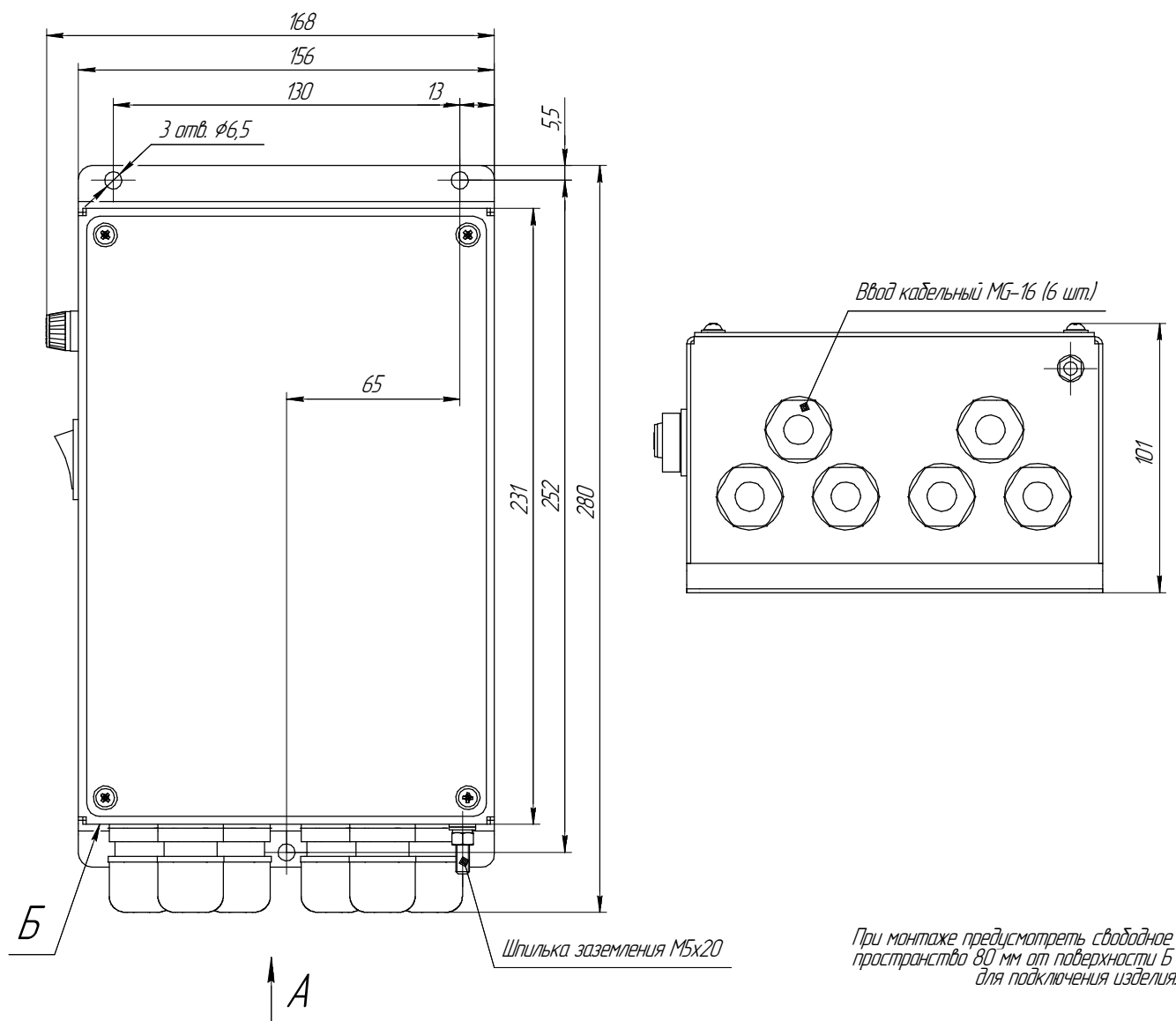
Габаритные и установочные размеры БП-103
