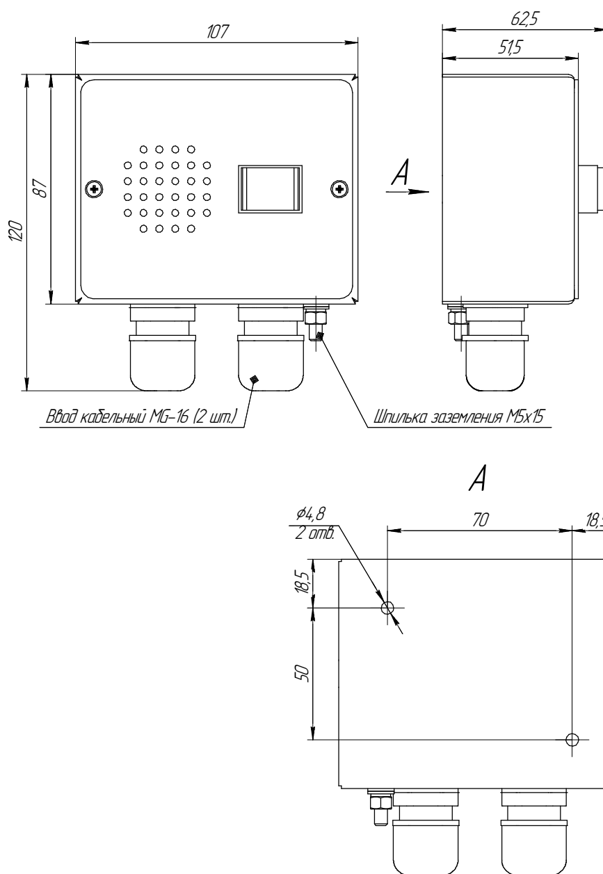
Габаритные и установочные размеры БС-106
