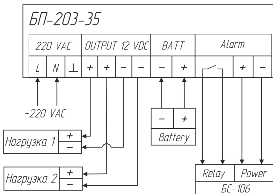
Рисунок 2 – Схема подключения изделия
