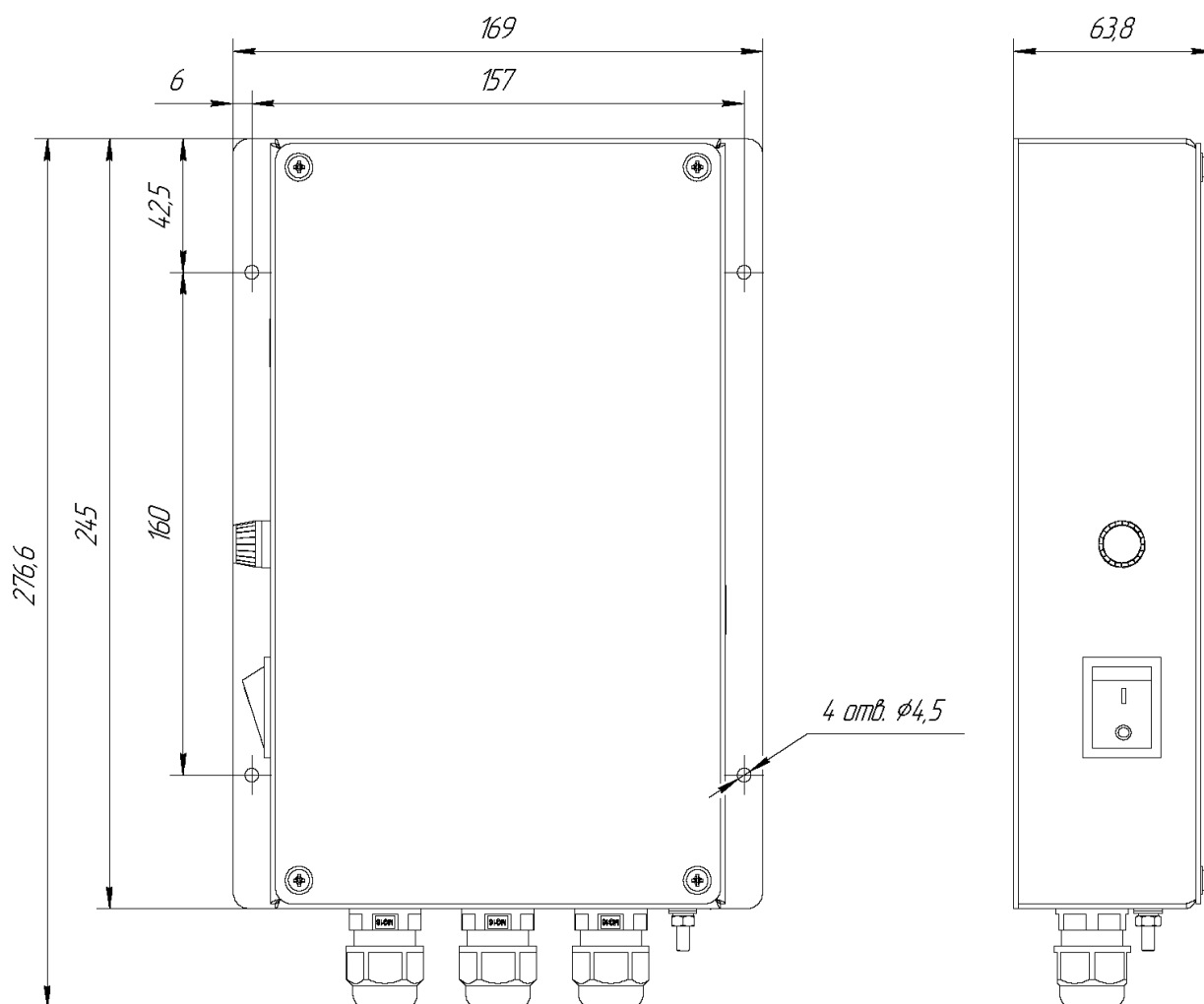
Рисунок Б.1 – Габаритные и установочные размеры изделия
