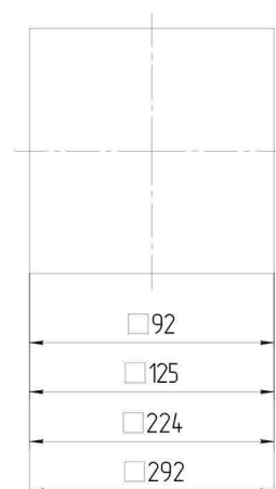
Монтажный вырез
