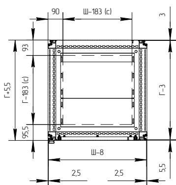
Б-Б
