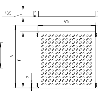
2916.xx Полка для 19" стационарная
