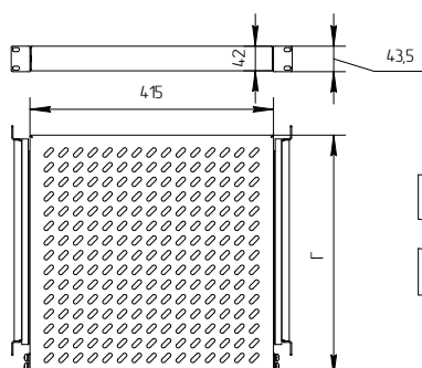
2915.xx Полка для 19" выдвижная
