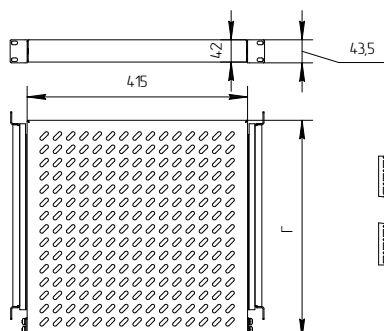
2915.xx Полка для 19" выдвижная
